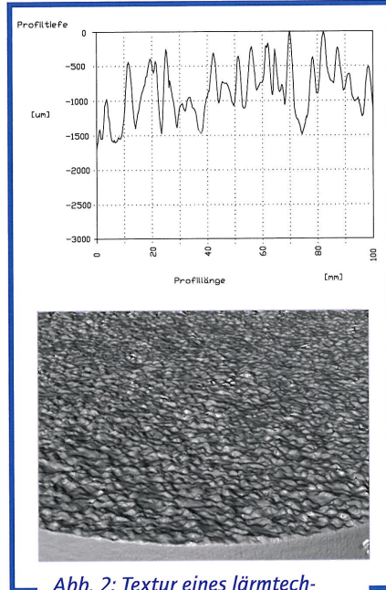
Abb. 2: Textur eines lärmtechnisch optimierten Gussasphaltes MA 5 S LA im Laserscan*
