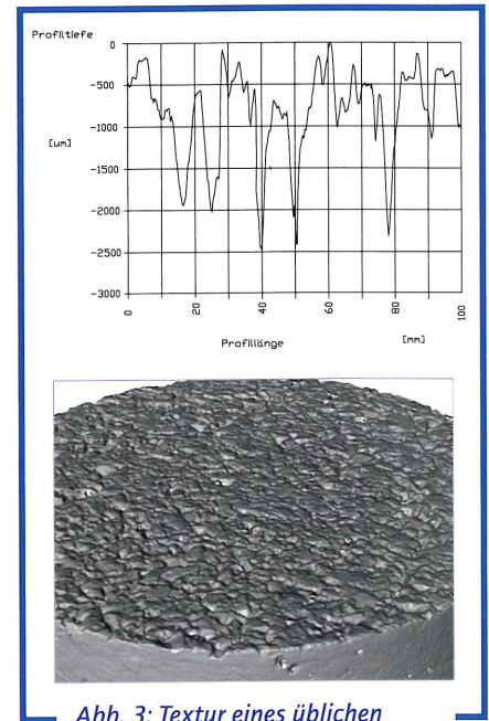
Abb. 3: Textur eines üblichen Splittmastixbelages SMA 11 S (ohne Abstumpfung) im Laserscan*
