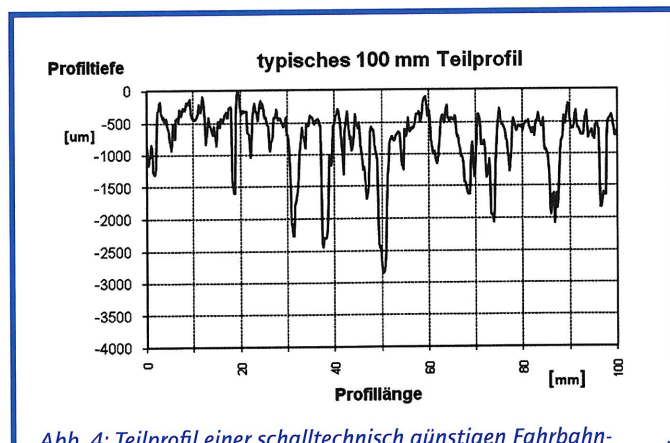
Abb. 4: Teilprofil einer schalltechnisch günstigen Fahrbahn-deckschicht aus lärmtechnisch optimierten Dünnschichtbelages DSH-V 0/5 LA
