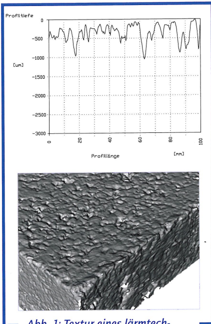
Abb. 1: Textur eines lärmtechnisch optimierten Dünnschichtbelages DSH-V 0/5 LA
